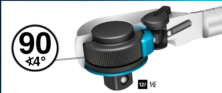
90 Zähne, 4° Schwenkwinkel
