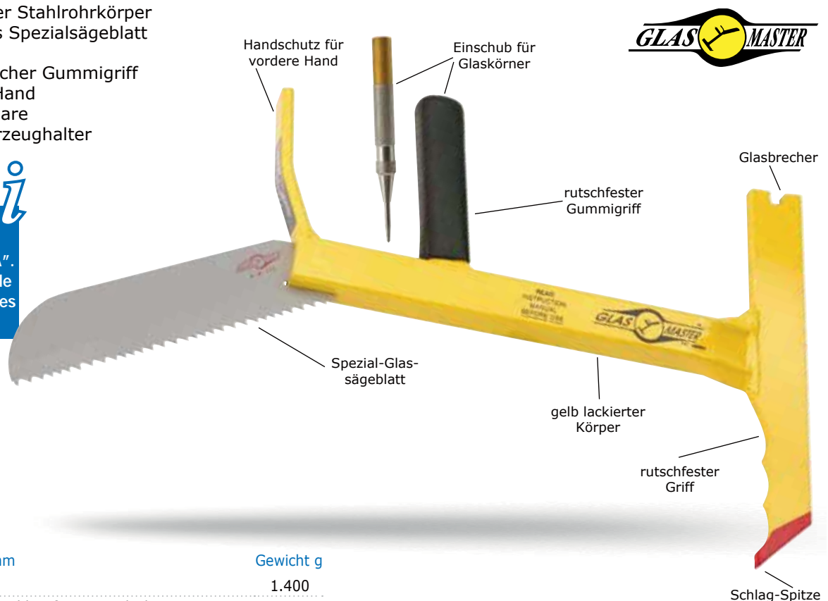
Einfaches und sicheres Brechen der Seitenscheiben mit dem Glasbrecher.
