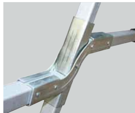
Zusätzliche Verstärkungen im Beinbereich.
